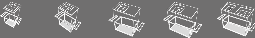
Era 48 Struttura sospesa Wall-hung framework cm 48 x 46 x 40 h Era 60 Struttura sospesa Wall-hung framework cm 60 x 46 x 40 h Era 80 Struttura sospesa Wall-hung framework cm 80 x 46 x 40 h Era 100 Struttura sospesa Wall-hung framework cm 100 x 46 x 40 h Era 120 Struttura sospesa Wall-hung framework cm 120 x 46 x 40 h
