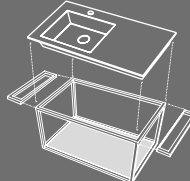
Era 80 Struttura sospesa Wall-hung framework cm 80 x 46 x 40 h
