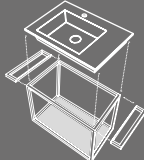
Era 60 Struttura sospesa Wall-hung framework cm 60 x 46 x 40 h
