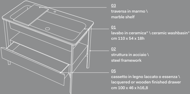
Catino Rettangolare con cassetto \ with drawer - cm 110 x 58,5 x h83
