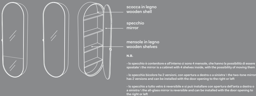
Elio Slim: dimensioni \ sizes - cm 140 x 50 x 12,8
